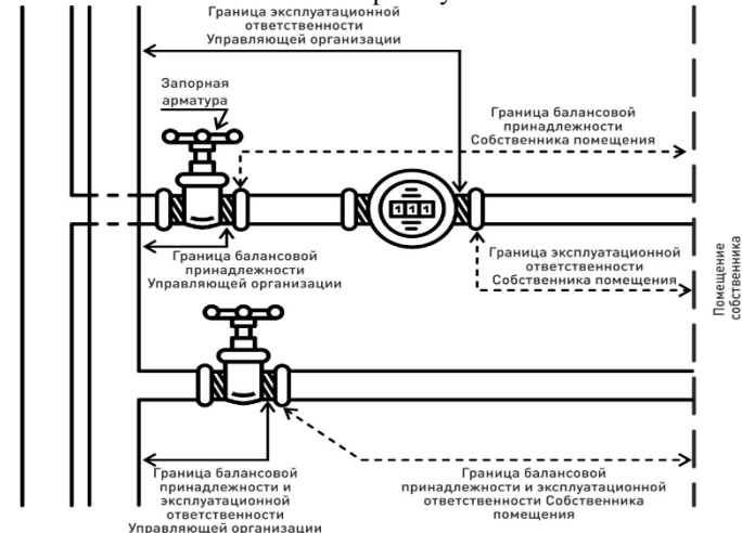
Схема №2. Граница балансовой принадлежности и эксплуатационной ответственности УО при лучевой разводке системы отопления в коллекторном узле
