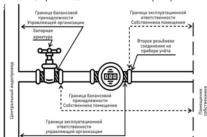
Схема №1. Граница балансовой принадлежности и эксплуатационной ответственности УО при лучевой разводке холодного, горячего водоснабжения в коллекторном узле.
